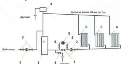
Схема открытой системы отопления
