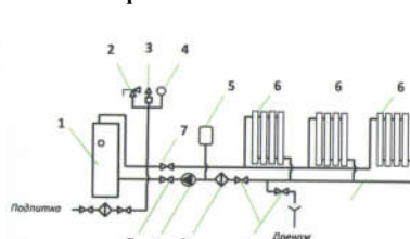
Схема закрытой системы отопления
